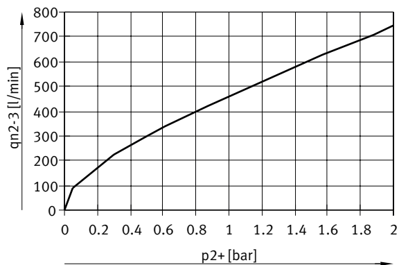
Durchfluss q_n von 2 → 3 in Abhängigkeit vom Ausgangsüberdruck p_2 , VPPM-8L/F-...-0L2H-... (2 bar)
