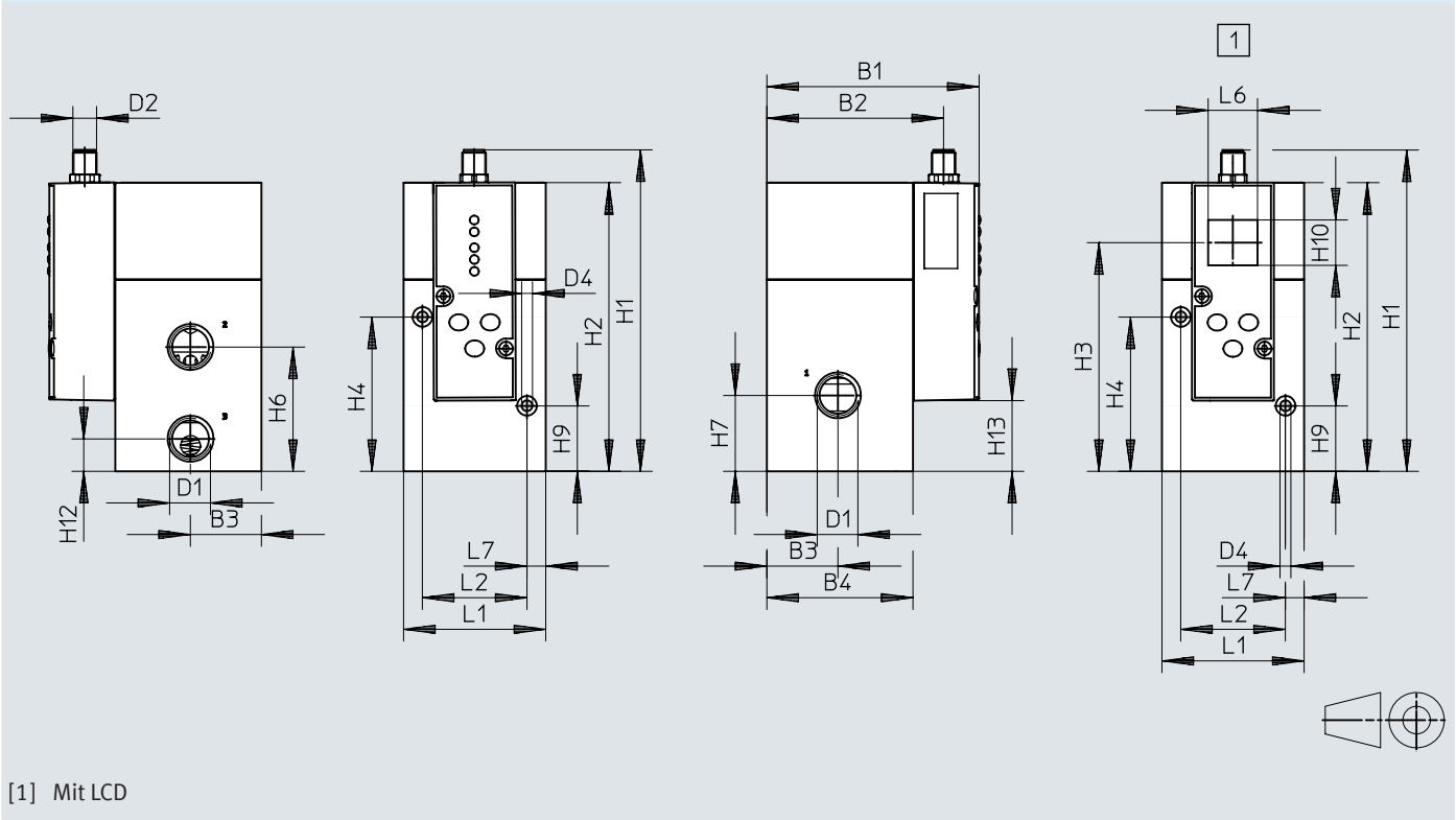
Abmessungen – VPPM-12L, mit LCD
