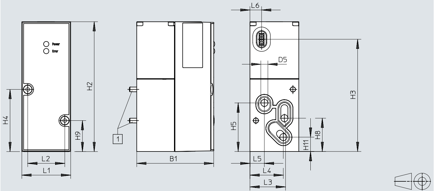
[1] Zylinderschraube M4x55
