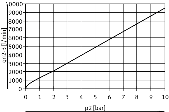
Durchfluss qn von 2 → 3 in Abhängigkeit vom Ausgangsüberdruck p2, VPPM-12L-...-0L10H-... (11 bar)
