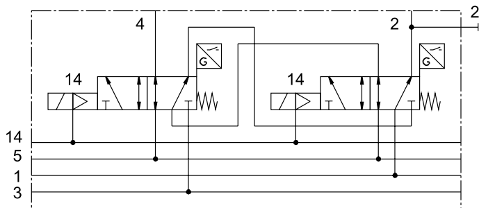
[5] 5/2-Wegeventil
