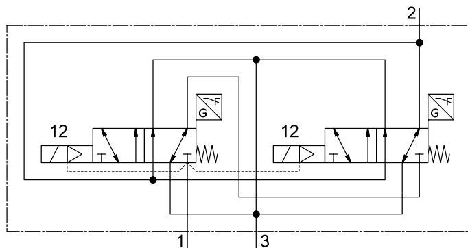
[3GL] 3/2-Wegeventil, Ruhestellung geschlossen
