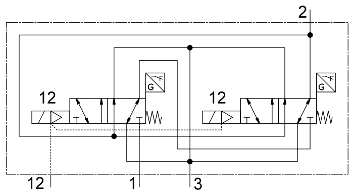
[M32C] 3/2-Wegeventil, Ruhestellung geschlossen
