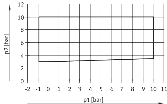
Steuerdruck p2 in Abhängigkeit vom Arbeitsdruck p1, für Tellersitz-Ventile VMEF-...-M32... (Ruhestellung geschlossen)
