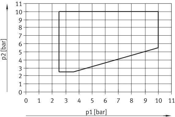
Steuerdruck p2 in Abhängigkeit vom externen Luftfederdruck p1, für Kolbenschieber-Ventile VMEF-...-M52...14
