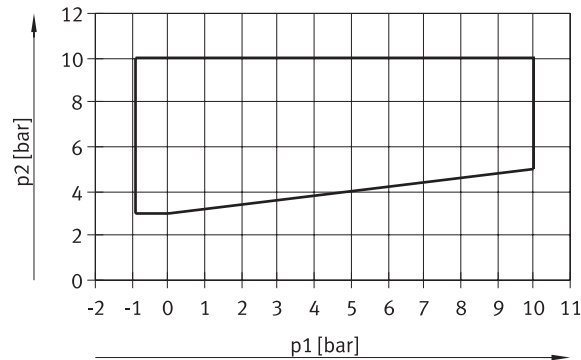
Steuerdruck p2 in Abhängigkeit vom Arbeitsdruck p1, für Tellersitz-Ventile VMEF-...-M32... (Ruhestellung offen)
