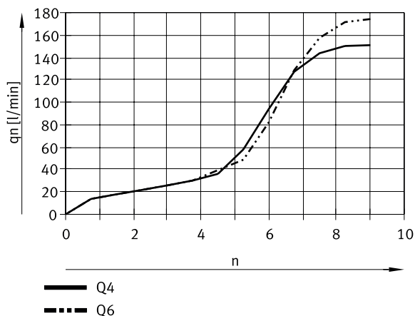
Normaldurchfluss q_n bei 0,6 → 0 MPa in Abhängigkeit der Spindelumdrehungen n für Gewindeanschluss M5 (Abluft)
