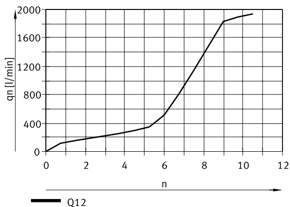
Normaldurchfluss q_n bei 0,6 → 0 MPa in Abhängigkeit der Spindelumdrehungen n für Gewindeanschluss G1/2, R1/2 (Abluft)
