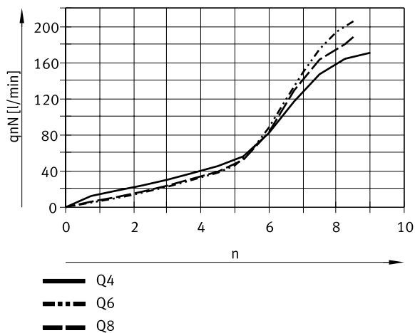
Normalnennendurchfluss q_{nN} bei 0,6 → 0,5 MPa in Abhängigkeit der Spindelumdrehungen n für Gewindeanschluss G1/8, R1/8 (Abluft)
