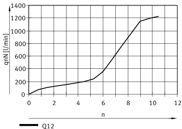
Normalnennendurchfluss q_{nN} bei 0,6 → 0,5 MPa in Abhängigkeit der Spindelumdrehungen n für Gewindeanschluss G1/2, R1/2 (Abluft)
