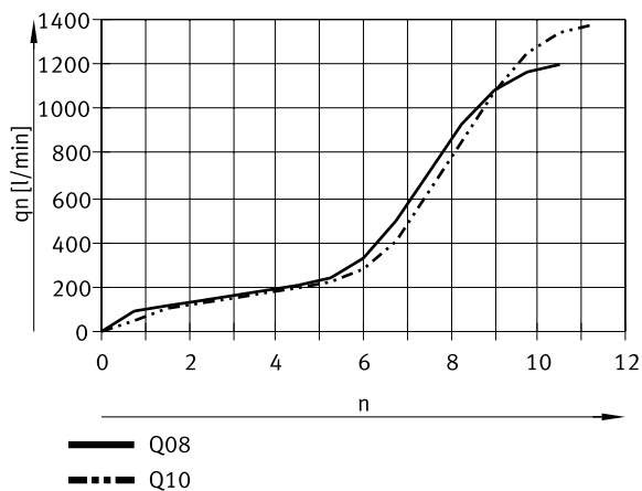
Normaldurchfluss q_n bei 0,6 → 0 MPa in Abhängigkeit der Spindelumdrehungen n für Gewindeanschluss G3/8, R3/8 (Abluft)
