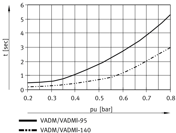
Evakuierungszeit t [s] für 1 Liter Volumen bei 6 bar Betriebsdruck (Nennweite Lavaldüse 95/140)
