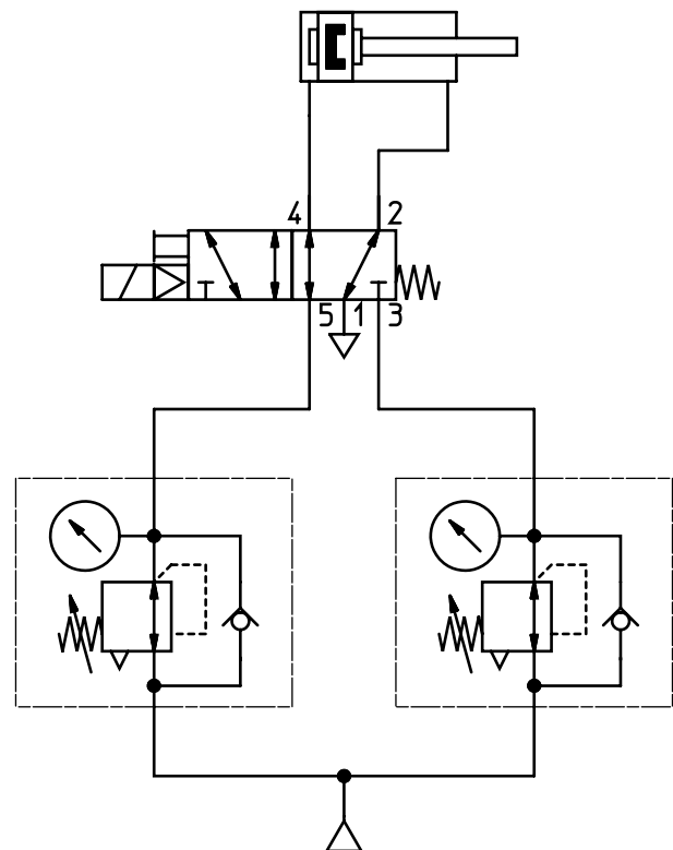
Zweidruckbetrieb mit reversiblen Regler
