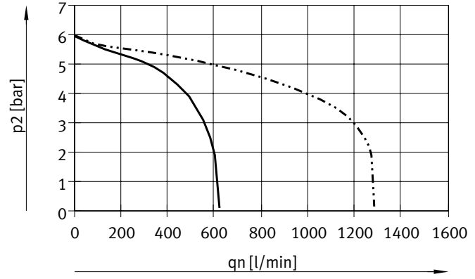
Durchfluss qn in Abhängigkeit vom Ausgangsdruck p2 mit Druckreglerplatten (P-Reglerplatte) für Anschluss 1
