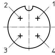
[1] Anschluss-Stecker M12x1, Stift, 4-polig nach EN 61076-2-101
