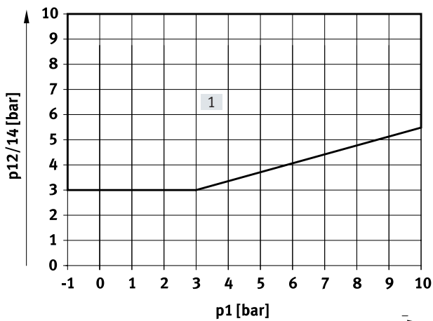
[1] Arbeitsbereich für Ventile mit externer Steuerluftversorgung
