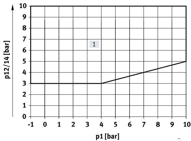
[1] Arbeitsbereich für Ventile mit externer Steuerluftversorgung
