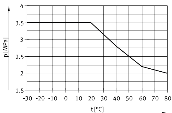
Betriebsdruck p in Abhängigkeit von der Temperatur t (Außen-Ø 4 ... 16 mm)
