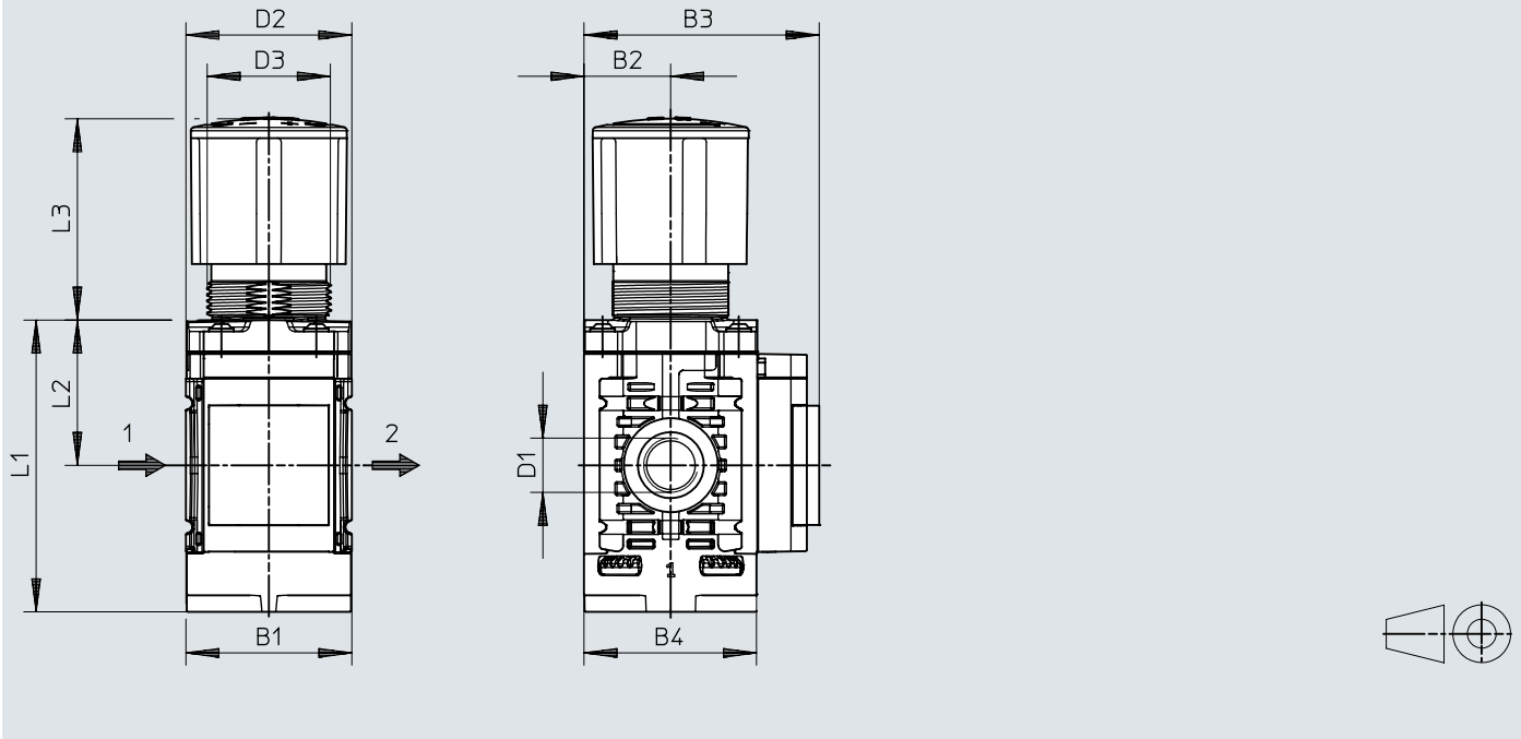
Abmessungen – MS4-LR mit Manometer
