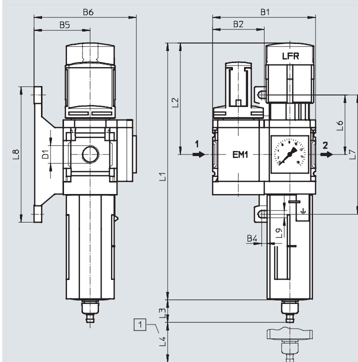
[1] Einbaumaß
