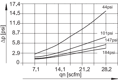
Differenzdruck \Delta p in Abhängigkeit vom Normaldurchfluss am Ausgang q_n (MS6N-LDM1-...-P40)
