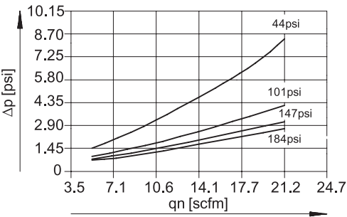
Differenzdruck \Delta p in Abhängigkeit vom Normaldurchfluss am Ausgang q_n (MS6N-LDM1-...-P30)
