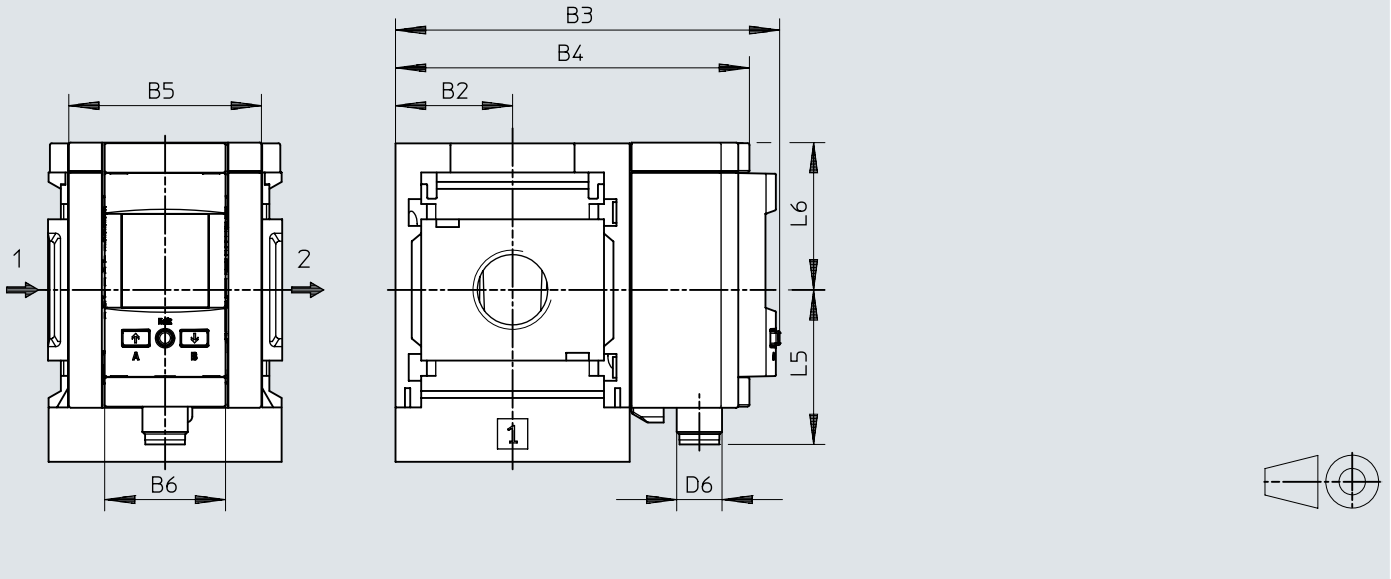
Abmessungen – AD11/AD12 Drucksensor mit LCD-Anzeige
