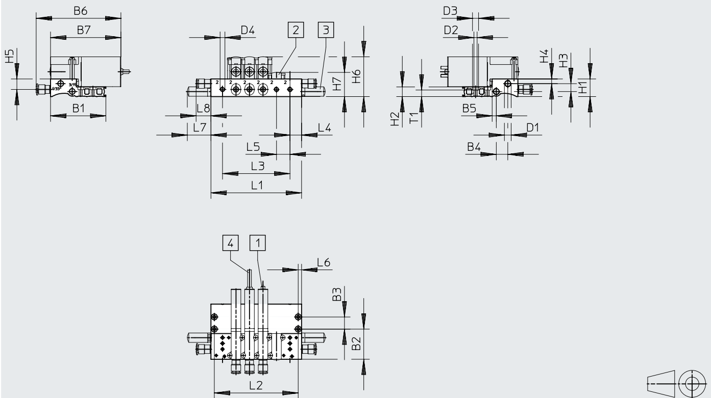
[1] Steckerfahnen [2] Abdeckplatte [3] Schalldämpfer [4] Kabel 2,5 m
