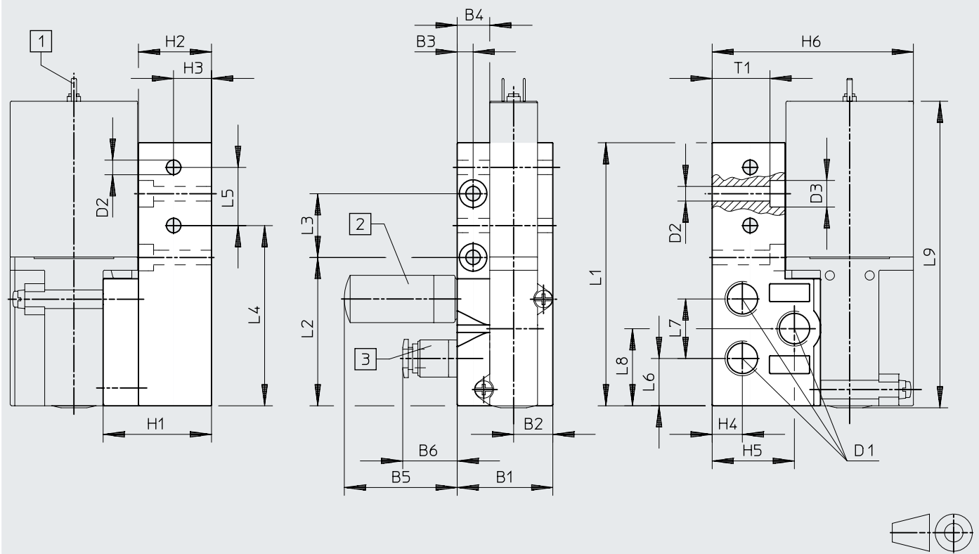
[1] Steckerfahnen [2] Schalldämpfer [3] Steckverschraubung
