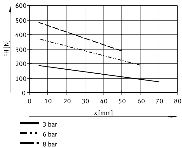
Greifkraft FH pro Greifbacken in Abhängigkeit vom Betriebsdruck und dem Hebelarm x – Außengreifen (schließen), doppelwirkend – HGDD-50
