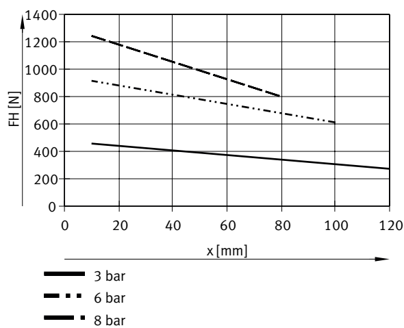
Greifkraft FH pro Greifbacken in Abhängigkeit vom Betriebsdruck und dem Hebelarm x – Außengreifen (schließen), doppelwirkend – HGDD-80
