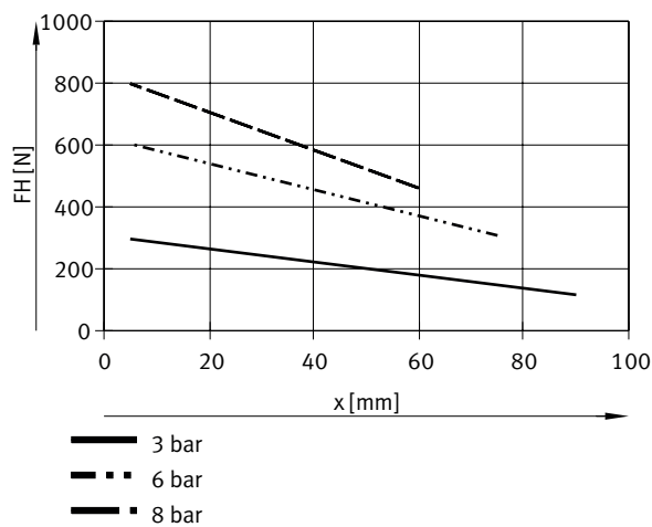
Greifkraft FH pro Greifbacken in Abhängigkeit vom Betriebsdruck und dem Hebelarm x – Außengreifen (schließen), doppelwirkend – HGDD-63
