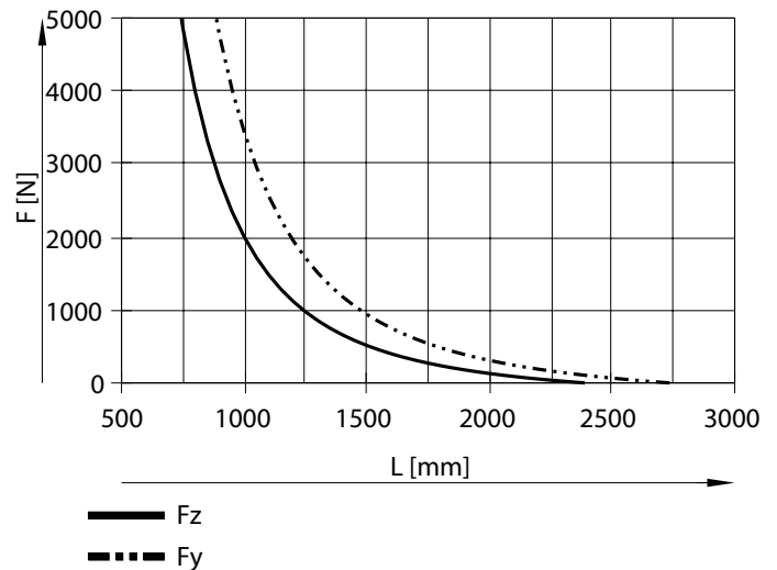
Baugröße 80
