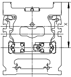
Abstand von Schlittenoberfläche zur Führungsmitte
