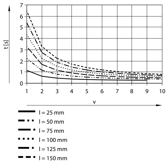
Positionierzeit t in Abhängigkeit von Geschwindigkeitsstufe v und Hub l mit Parallelbausatz für EGSS-BS-45
