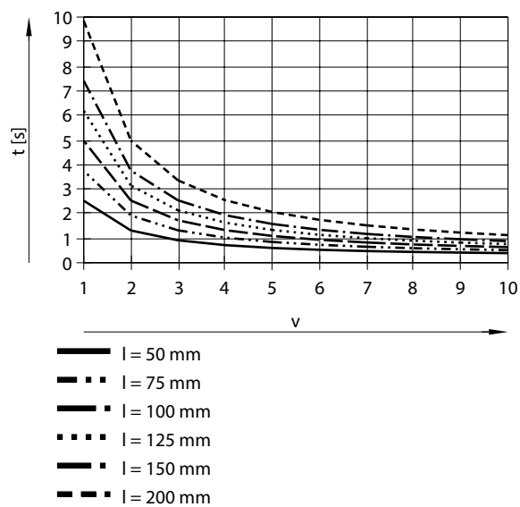
Positionierzeit t in Abhängigkeit von Geschwindigkeitsstufe v und Hub l mit Parallelbausatz für EGSS-BS-60
