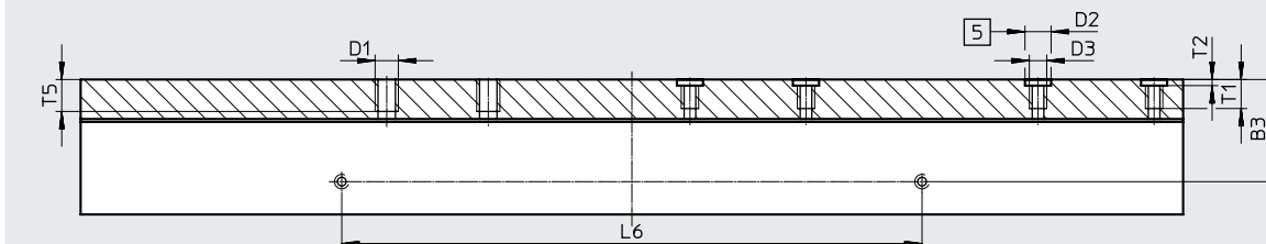
Ansicht A
