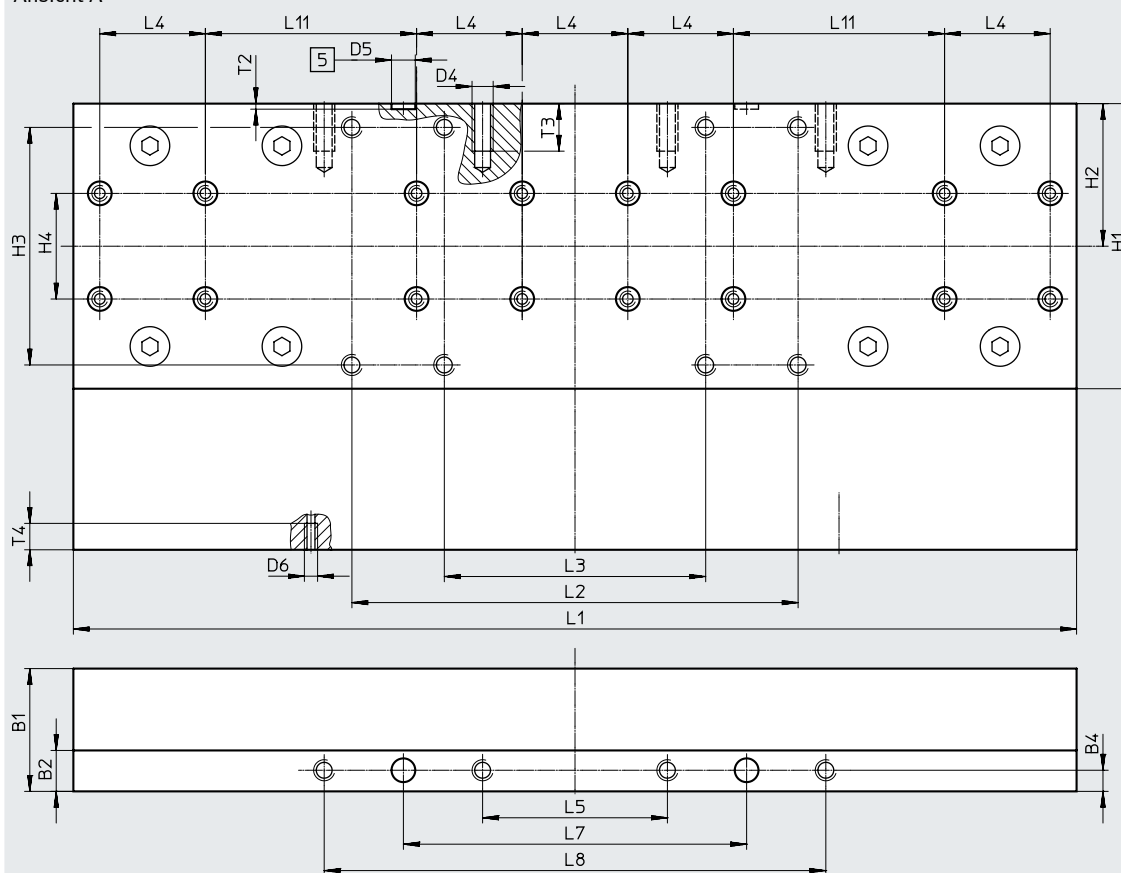
Ansicht A
