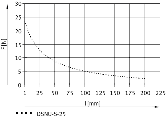
Max. Querkraft F_q in Abhängigkeit von Auskragung l – DSNU-S-25
