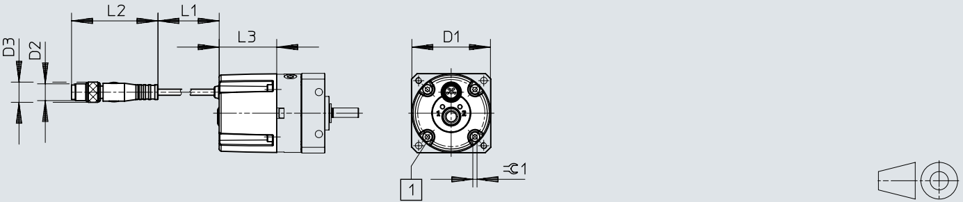
[1] Befestigungsschraube
