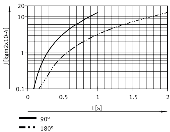
Massenträgheitsmoment J in Abhängigkeit von der Schwenkzeit t – DRVS-8
