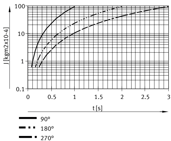
Massenträgheitsmoment J in Abhängigkeit von der Schwenkzeit t – DRVS-16
