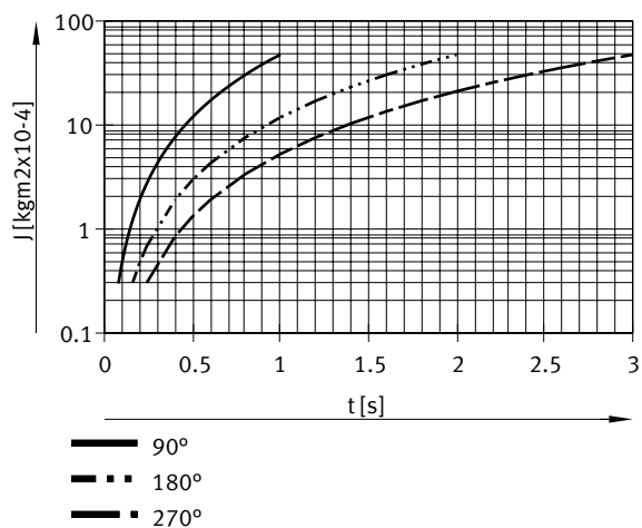
Massenträgheitsmoment J in Abhängigkeit von der Schwenkzeit t – DRVS-12
