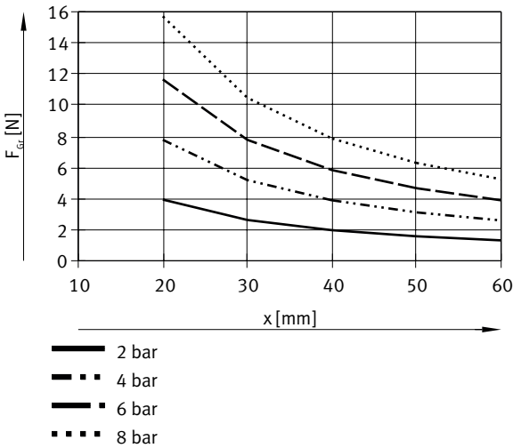
Greifkraft F pro Greifbacken in Abhängigkeit vom Betriebsdruck und dem Hebelarm x – Innengreifen (öffnen), doppelwirkend – DHWC-10-A
