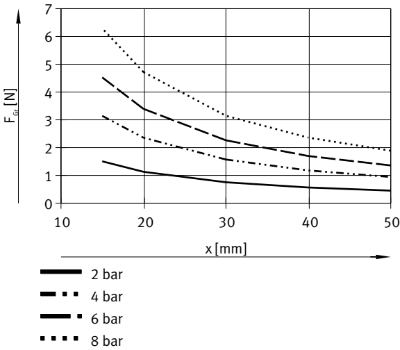
Greifkraft F pro Greifbacken in Abhängigkeit vom Betriebsdruck und dem Hebelarm x – Innengreifen (öffnen), doppelwirkend – DHWC-6-A
