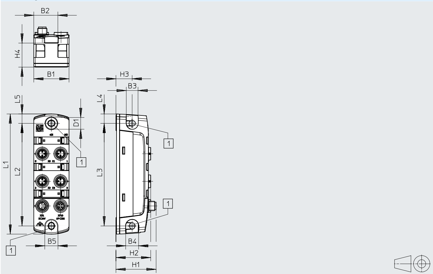
[1] Befestigungsbohrung für Schrauben M4
