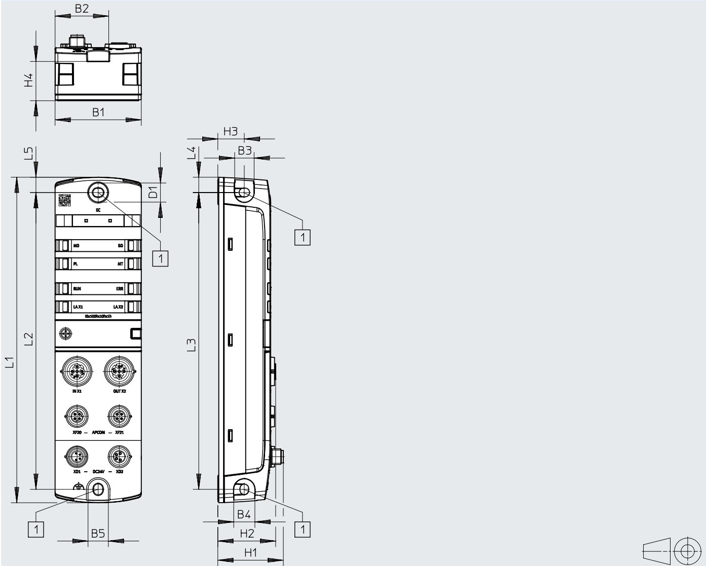
[1] Befestigungsbohrung für Schrauben M4
