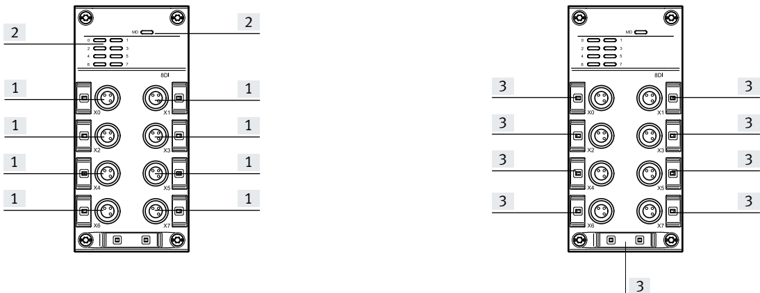
[1] Elektrischer Anschluss Eingänge [2] LED-Anzeigen [3] Platz für Bezeichnungsschild
