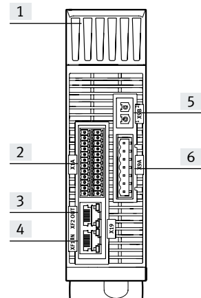
CMMT-AS-...-3A
