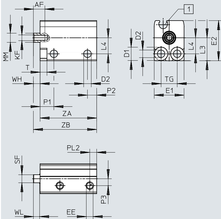
[1] Rundnut für Näherungsschalter
