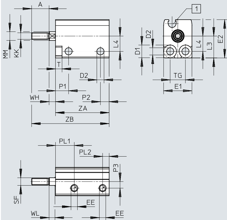
[1] Rundnut für Näherungsschalter
