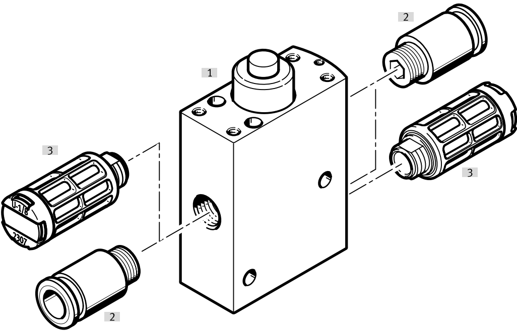
Cuadro general de periféricos, válvula accionada por leva 3/2
