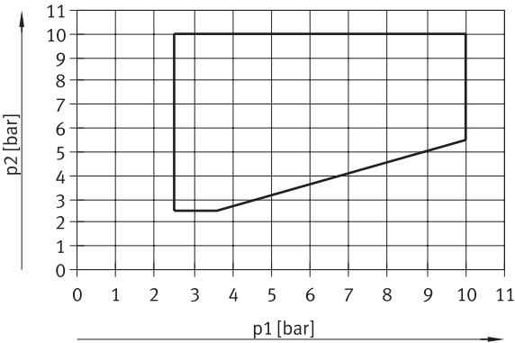
Presión de mando p2 en función de la presión externa del muelle neumático p1, para válvulas de corredera VMEF-...-M52...14
