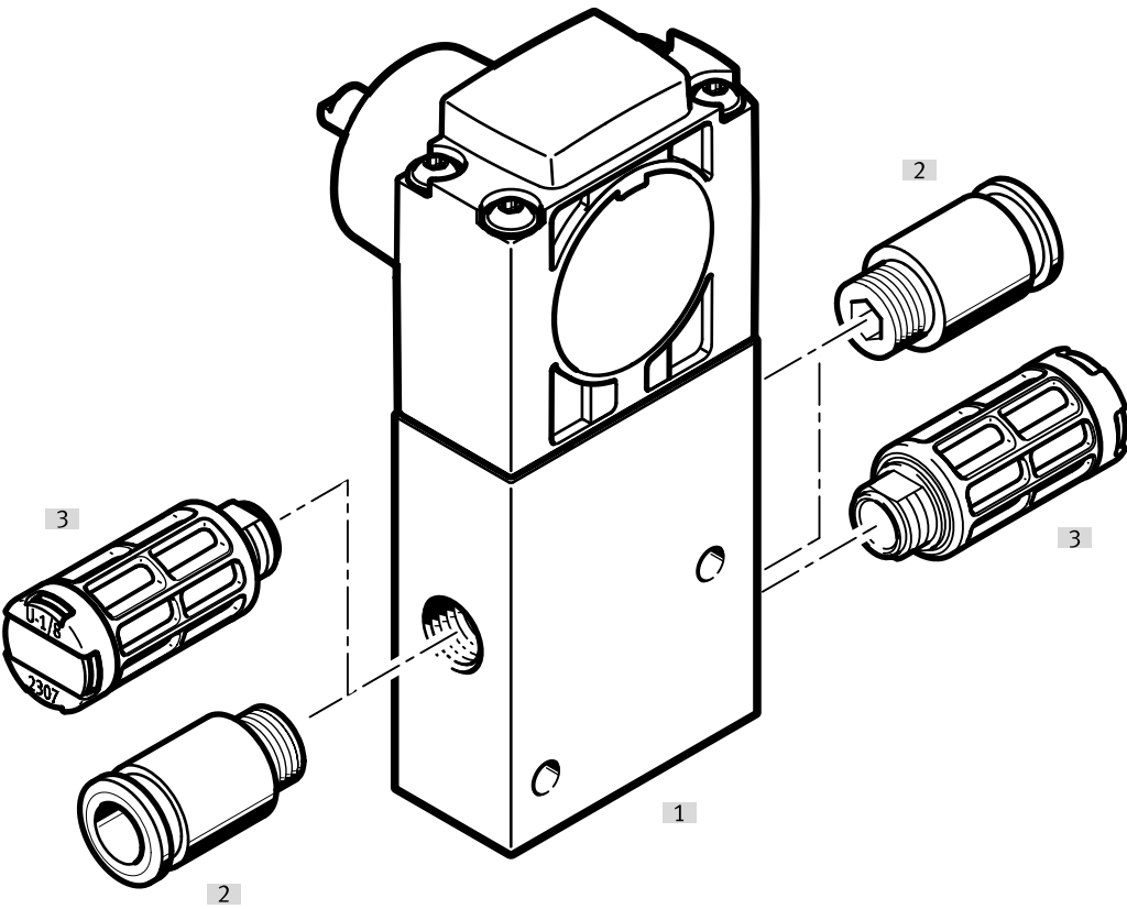
Cuadro general de periféricos, válvula de palanca giratoria 3/2
