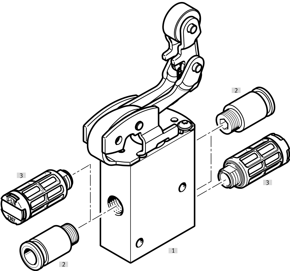
Cuadro general de periféricos, válvula de palanca con rodillo abatible 3/2
