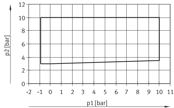
Presión de mando p2 en función de la presión de trabajo p1, para válvulas de asiento VMEF-...-M32... (normalmente cerrada)
