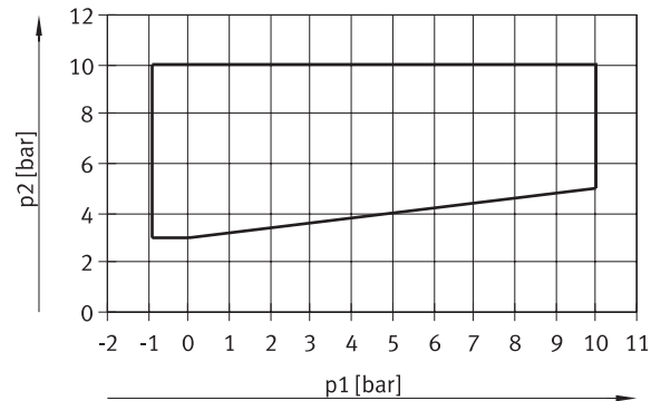
Presión de mando p2 en función de la presión de trabajo p1, para válvulas de asiento VMEF-...-M32... (normalmente abierta)
