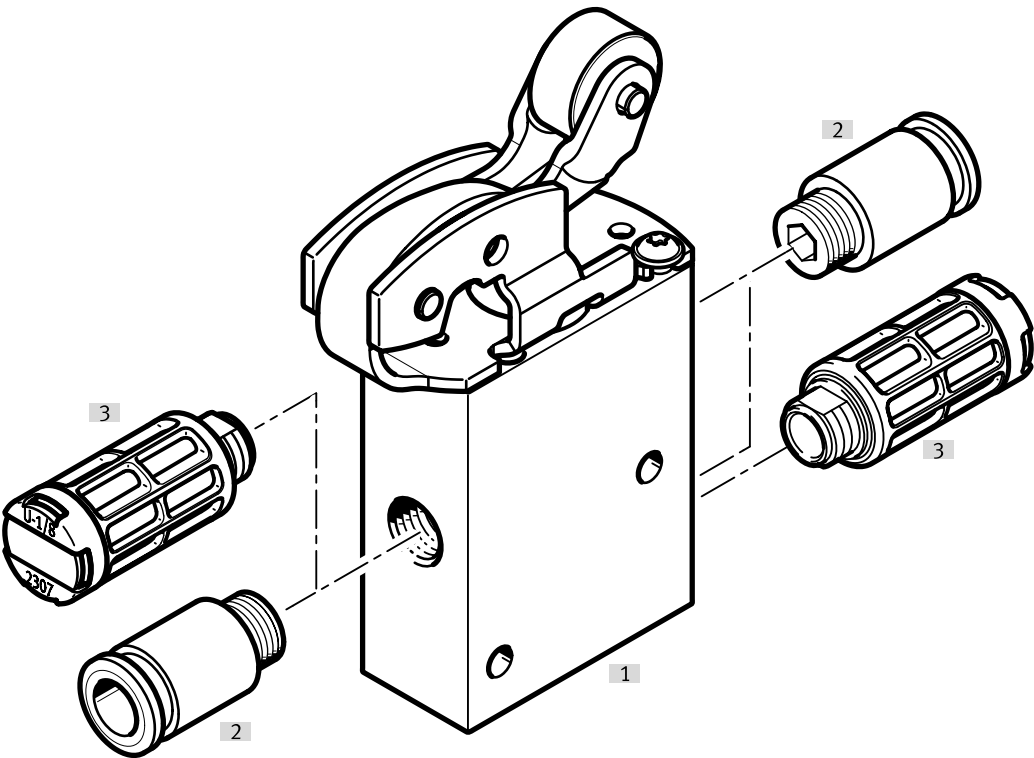
Cuadro general de periféricos, válvula de palanca de rodillo 3/2
