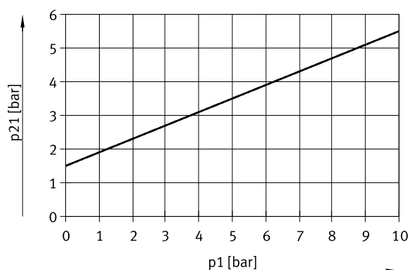
Presión mínima de mando p_{21} en función de la presión de funcionamiento p_1
