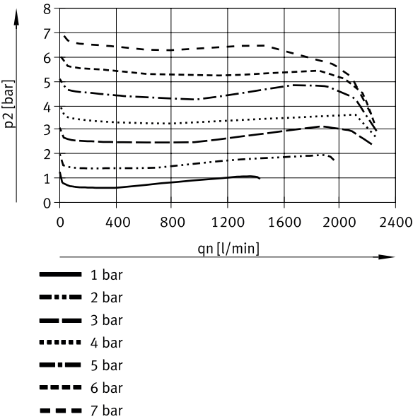
Caudal normal qn en función de la presión de salida p2 (p1 = 10 bar) – MS4-LFR...-C...-B (grado de filtración: 5 µm)
