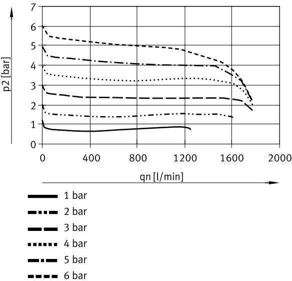
Caudal normal qn en función de la presión de salida p2 (p1 = 7 bar) – MS4-LFR...-E...-B (grado de filtración: 40 µm)
