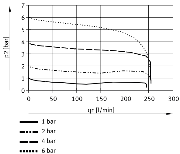
Caudal normal q_n en función de la presión de salida p_2 ( p_1 = 7 bar) – MS2-LFR-QS6-...-B (grado de filtración: 5\ \mu\text{m} )
