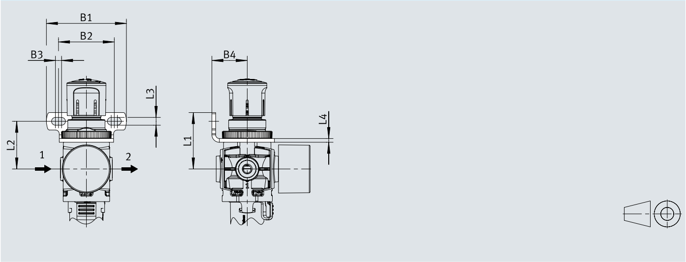
Dimensiones – Escuadra de fijación MS...-WR-B
