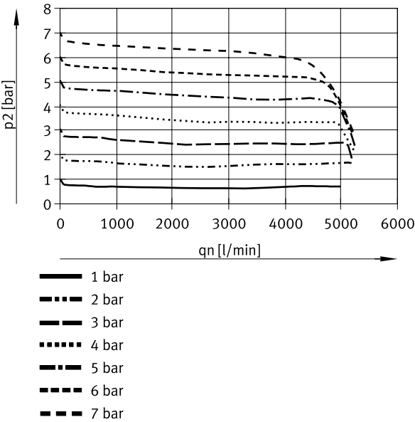
Caudal normal qn en función de la presión de salida p2 (p1 = 10 bar) – MS6-LFR...-C...-B (grado de filtración: 5 µm)
