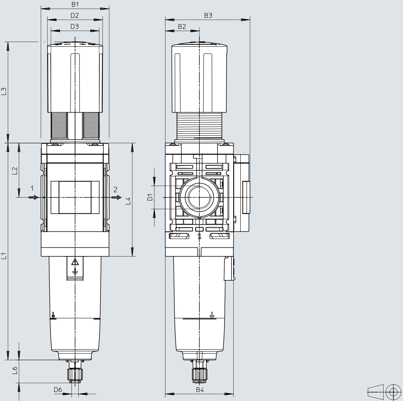
Dimensiones – MS6-LFR-...-B con manómetro
