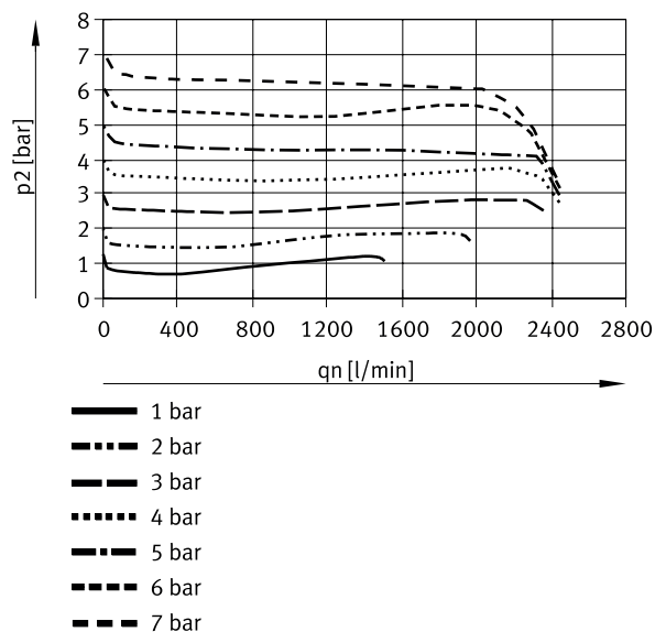
Caudal normal q_n en función de la presión de salida p_2 ( p_1 = 10 bar) – MS4-LFR...-E...-B (grado de filtración: 40 \mu\text{m} )
