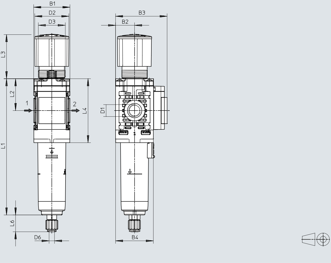
Dimensiones – MS4-LFR-...-B con manómetro
