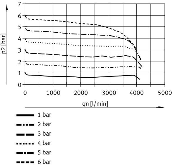
Caudal normal qn en función de la presión de salida p2 (p1 = 7 bar) – MS6-LFR...-E...-B (grado de filtración: 40 µm)
