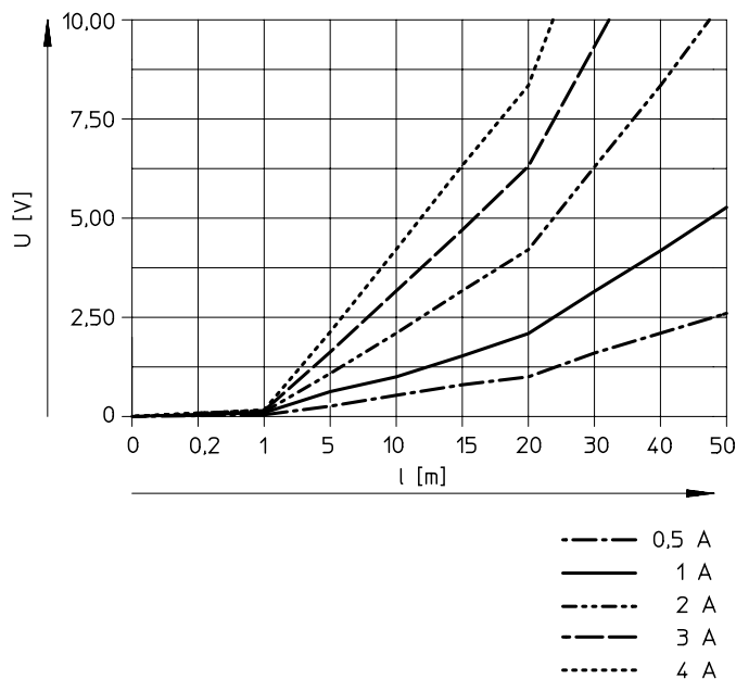
Caída de tensión U con sección de cable de 0,34 mm 2 con M12
