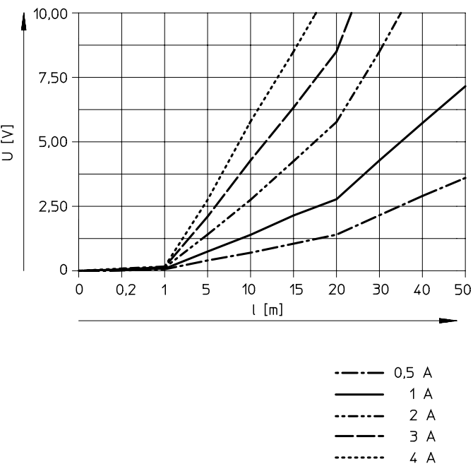
Caída de tensión U con sección de cable de 0,25 mm 2 con M12
