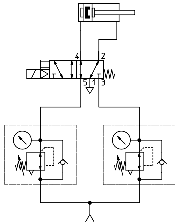
Zweidruckbetrieb mit reversiblem Regler
