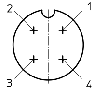
[1] Anschluss-Stecker M12x1, Stift, 4-polig nach EN 61076-2-101
