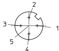
[1] Anschlussstecker M12x1, Stift, 5-polig
