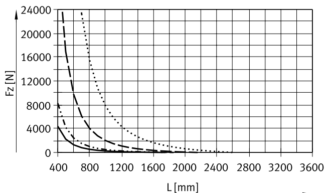
Kraft F_z
