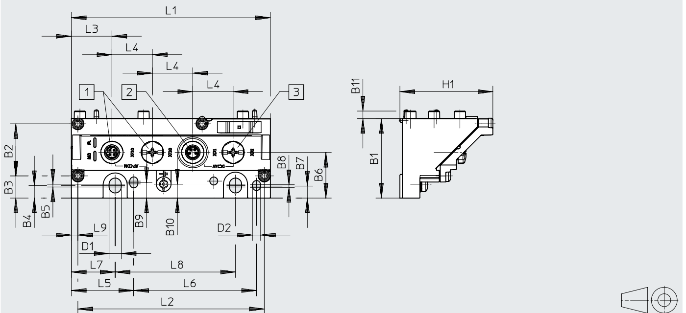
[1] Dose M8x1, D-codiert
