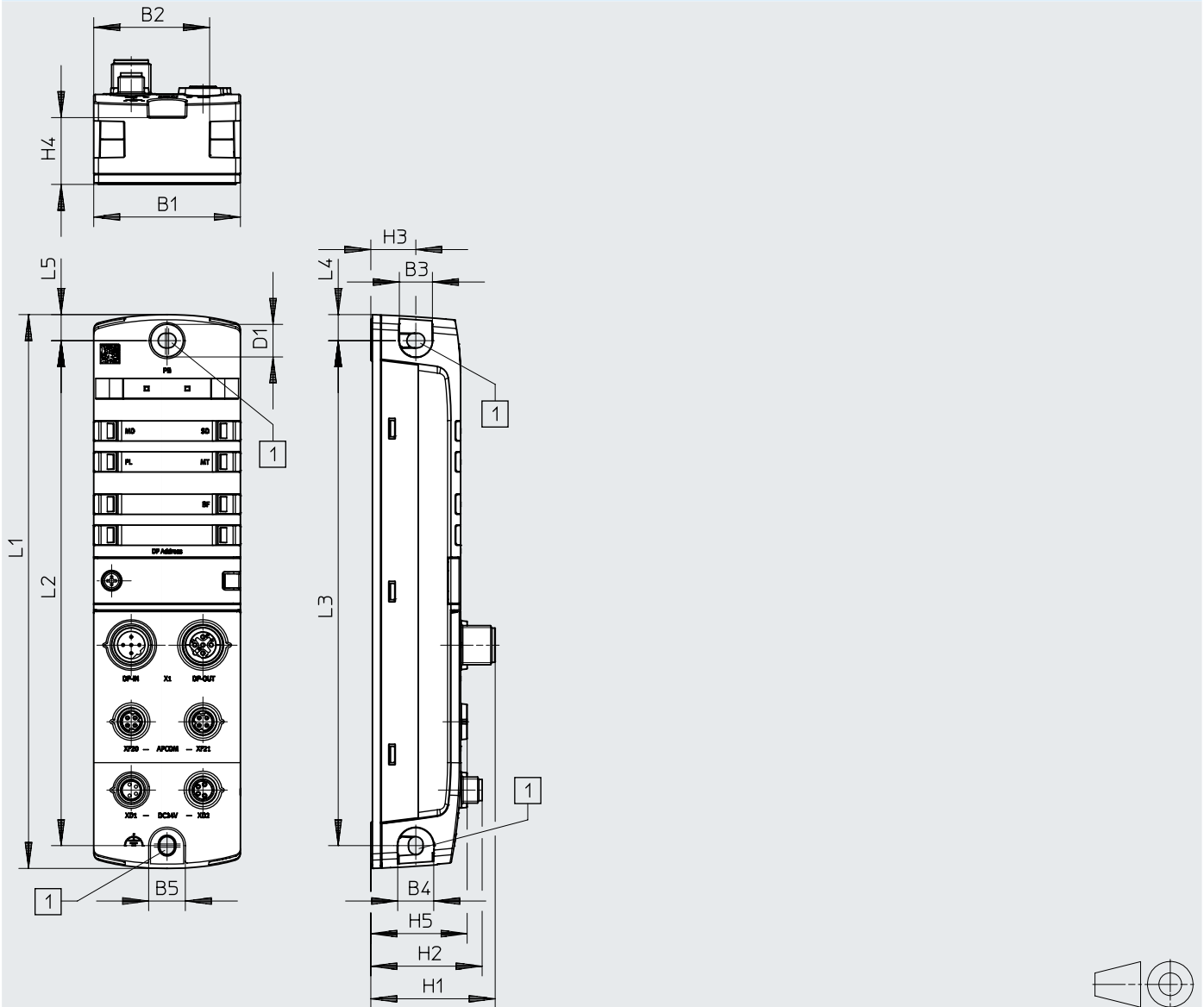
[1] Befestigungsbohrung für Schrauben M4
