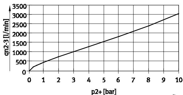
Débit q_n de 2 → 3 en fonction de la pression de sortie p_2
