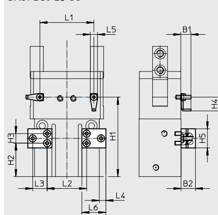
DASI-B10-25-S8
