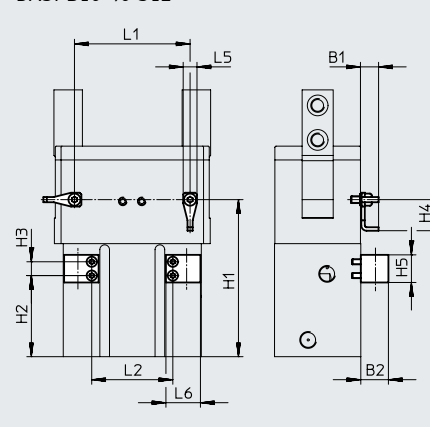
DASI-B10-40-S12
