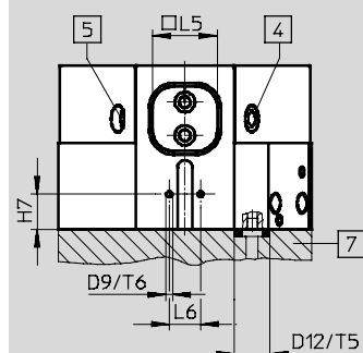
Vue A
