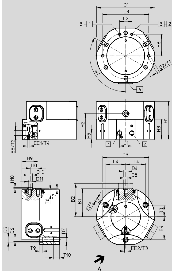
Vue A
