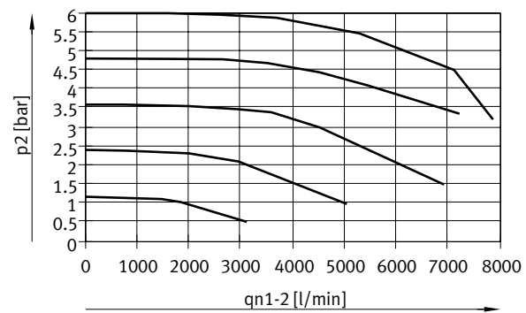
Caudal normal qn de 1 → 2 en función de la sobrepresión en la salida p2 VPPM-12L-...-0L2H-... (4 bar) VPPM-12L-...-0L6H-... (8 bar)
