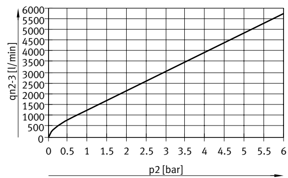
Caudal normal qn de 2 → 3 en función de la sobrepresión en la salida p2 VPPM-12L-...-0L2H-... (4 bar) VPPM-12L-...-0L6H-... (8 bar)
