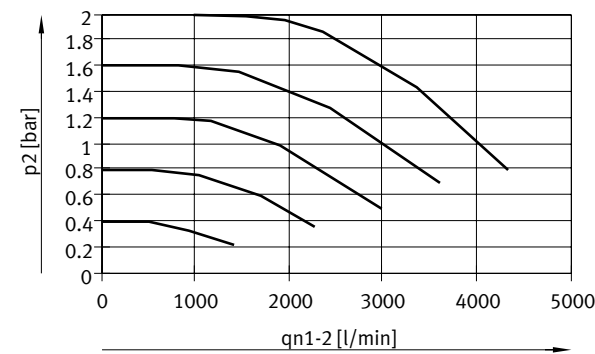
VPPM-12L-...-0L10H-... (11 bar)
