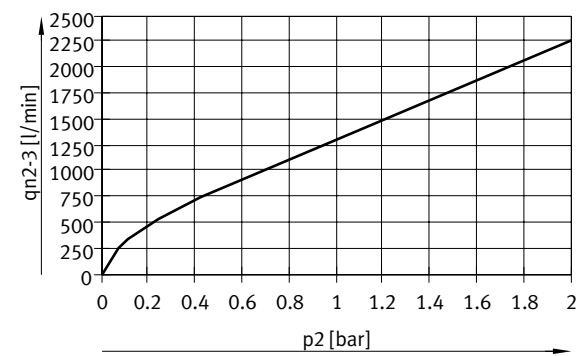
VPPM-12L-...-0L10H-... (11 bar)
