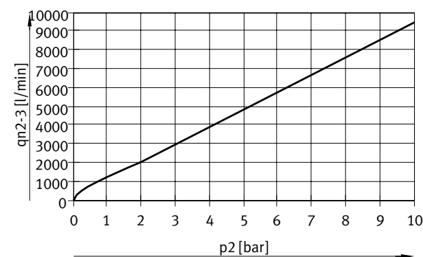
VPPM-12L-...-0L10H-... (11 bar)
