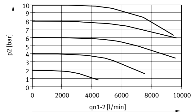
VPPM-12L-...-0L10H-... (11 bar)
