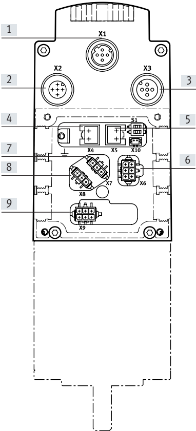
EMCA-...-CO
