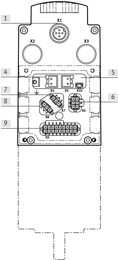
EMCA-...-DIO
