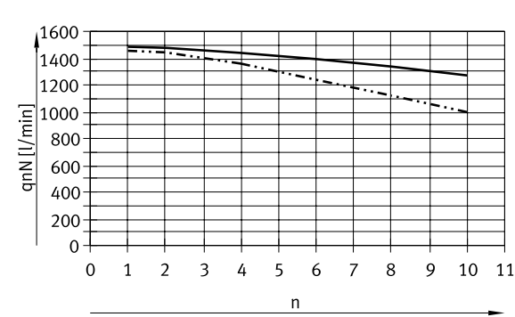
Para válvulas de 5/2 vías, sentido de flujo 1 → 4
