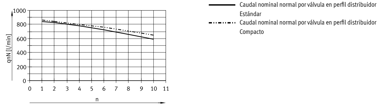
Para válvulas de 5/2 vías, sentido de flujo 1 → 2
