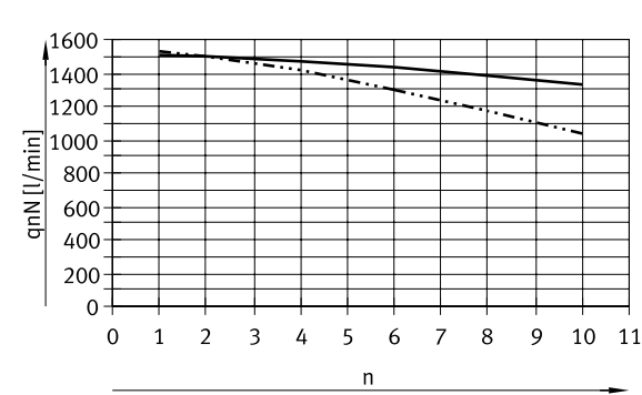
Para válvulas de 5/2 vías, sentido de flujo 1 → 2
