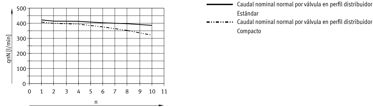
Para válvulas de 5/2 vías, sentido de flujo 1 → 4
