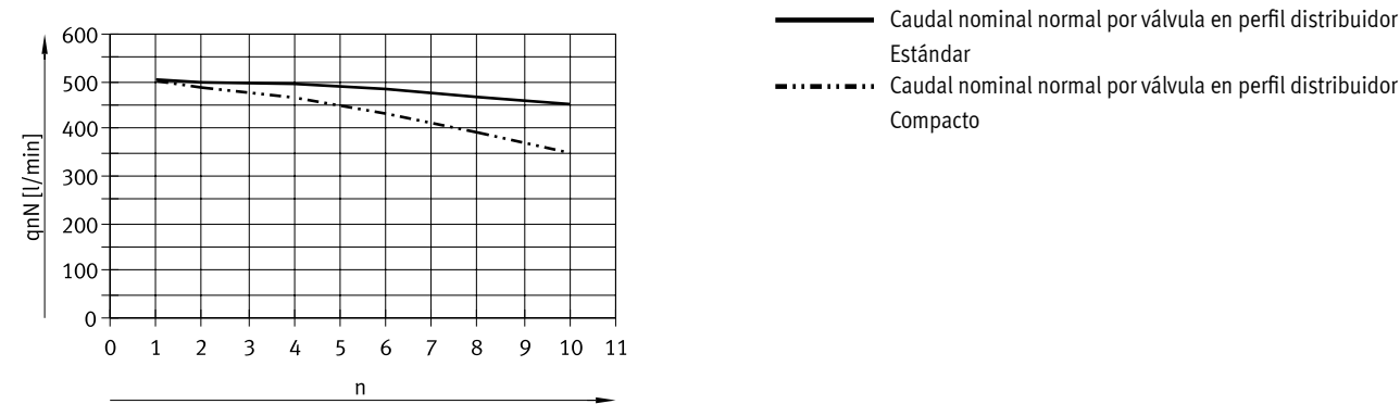
Para válvulas de 5/2 vías, sentido de flujo 1 → 2
