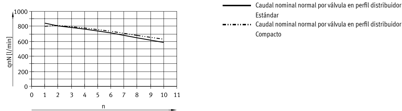
Para válvulas de 5/2 vías, sentido de flujo 1 → 4
