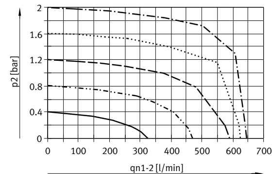
Caudal qn para válvulas con margen de regulación de la presión 0 ... 2 bar Sentido de flujo 1 > 2 en función de la presión de salida p2
