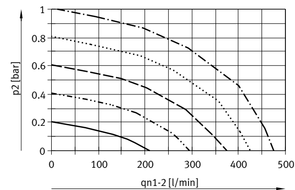
Caudal qn para válvulas con margen de regulación de la presión -1 ... +1 bar Sentido de flujo 1 > 2 en función de la presión de salida p2
