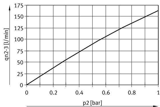
Sentido de flujo 2 > 3 en función de la presión de salida p2
