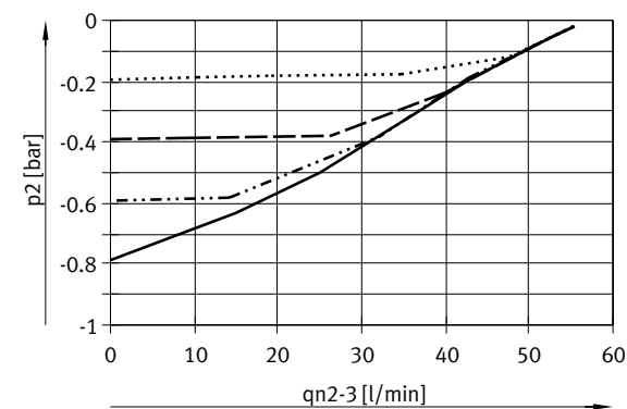
Caudal qn para válvulas con margen de regulación de la presión -1 ... 0 bar y para válvulas con margen de regulación de la presión -1 ... +1 bar Sentido de flujo 2 > 3 en función de la presión de salida p2
