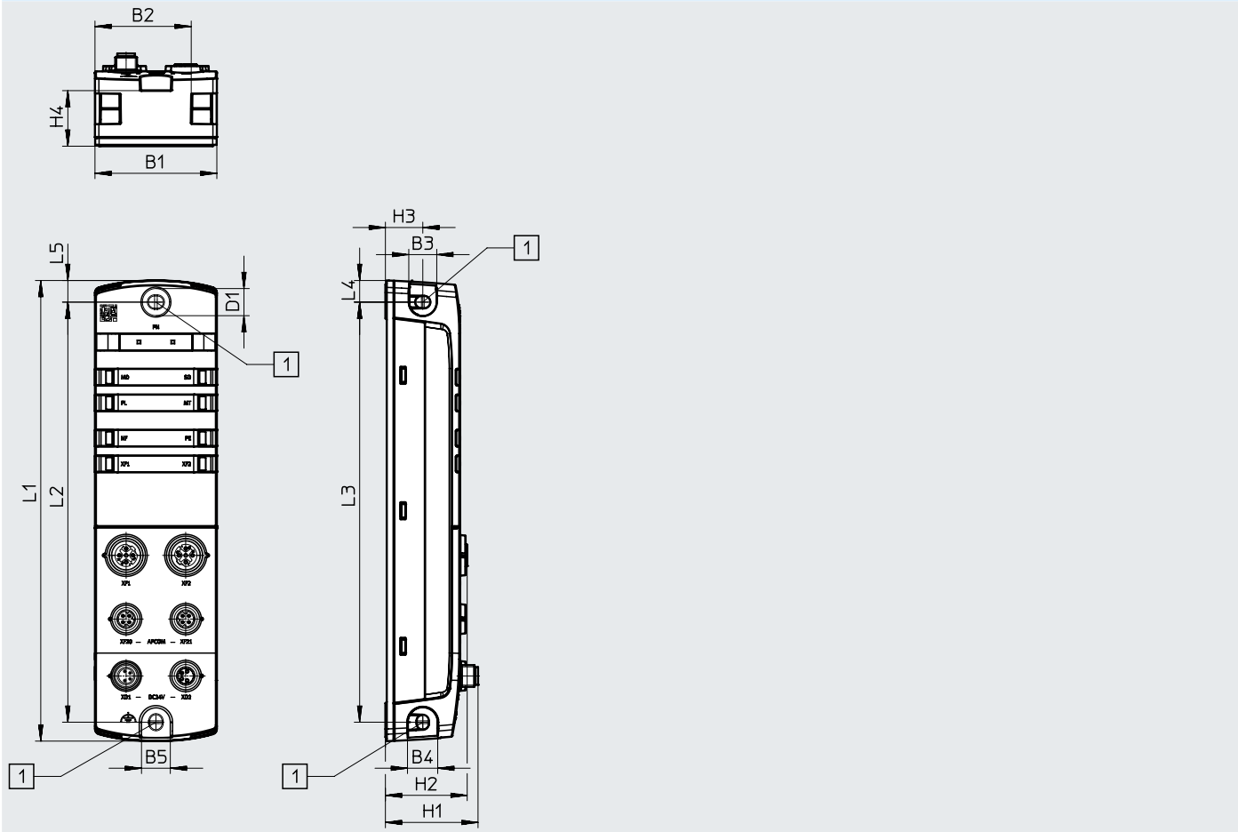
[1] Taladro de fijación para tornillos M4
