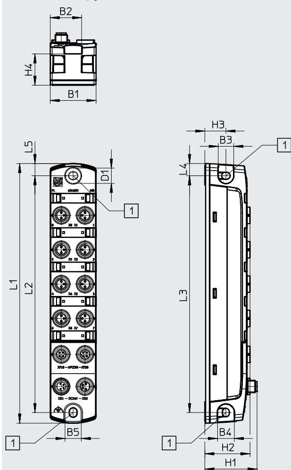
CPX-AP-I-4DI4DO-M8-3P
