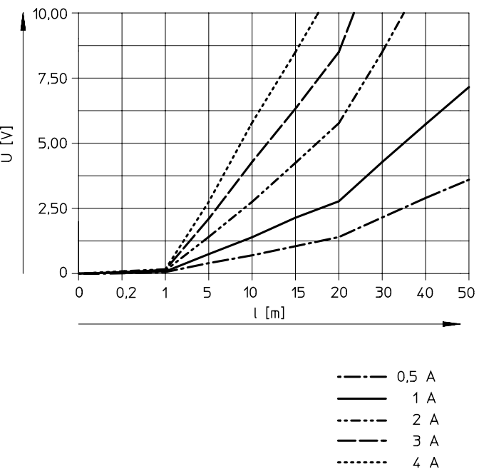
Caída de tensión U con sección de cable de 0,25 mm² con M12
