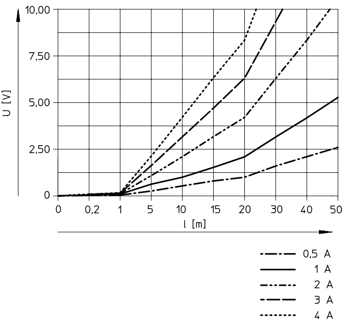
Caída de tensión U con sección de cable de 0,34 mm² con M12
