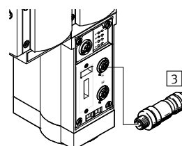
Feldbusknoten FB36 für EtherNet/IP, Feldbusknoten FB37 für EtherCAT
