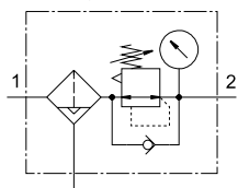
Kondensatablass halbautomatisch, mit Manometer
