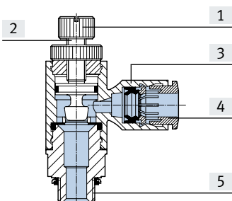
Drossel-Rückschlagventil
