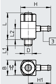
[3] Stecknippel
