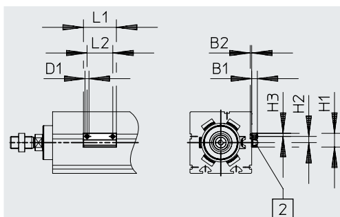
[2] Näherungsschalter
