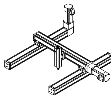
Portique tridimensionnel
