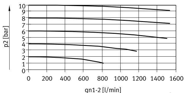
Caudal q_{n1-2} en función de la presión de salida p_2
