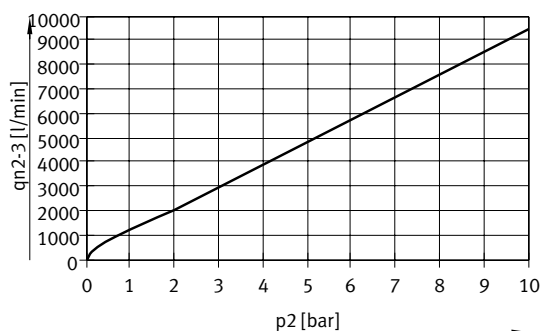
Caudal q_{n2-3} en función de la presión de salida p_2
