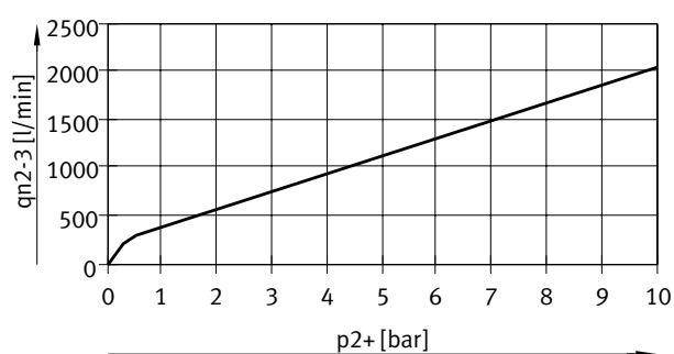
Caudal q_{n2-3} en función de la presión de salida p_2
