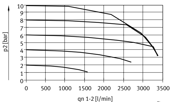
Caudal q_{n1-2} en función de la presión de salida p_2
