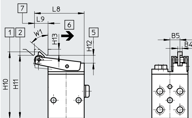
Válvula de palanca basculante LS-4-1/8
