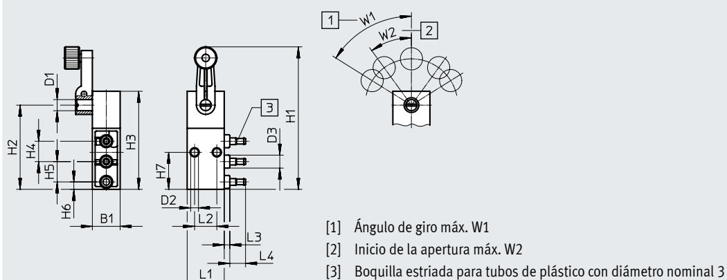
Válvula de palanca basculante RW/O-3-PK-3
