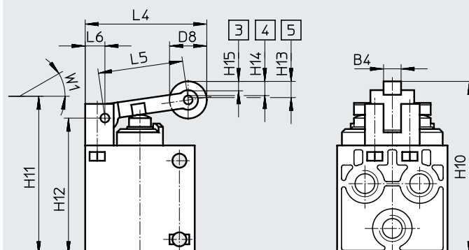
Válvula de palanca de rodillo R-5-1/4-B
