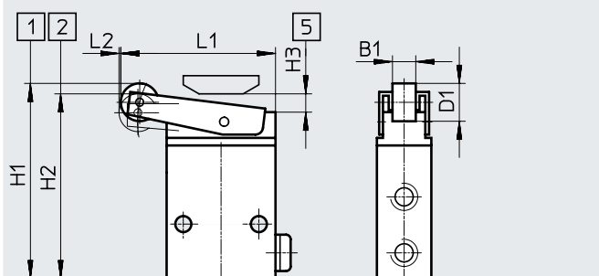
Válvula de palanca de rodillo RS-3-1/8, ROS-3-1/8
