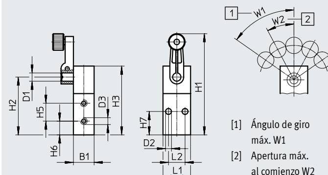
Válvula de palanca basculante RW-3-M5
