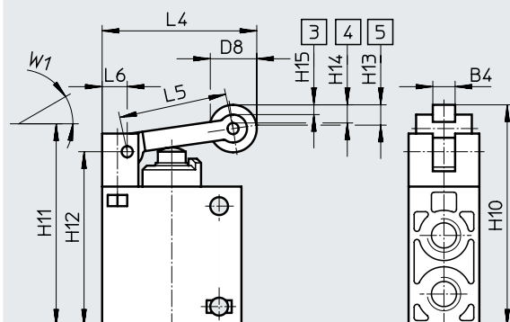
Válvula de palanca de rodillo R-3-1/4-B, R0-3-1/4-B
