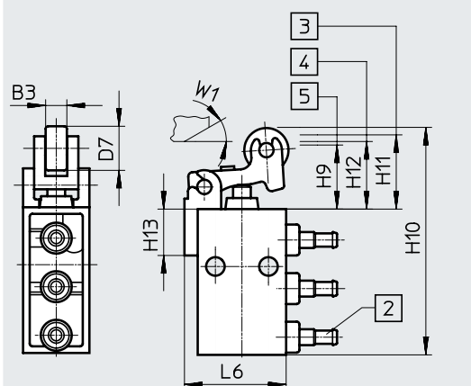
Válvula de palanca de rodillo R/O-3-PK-3
