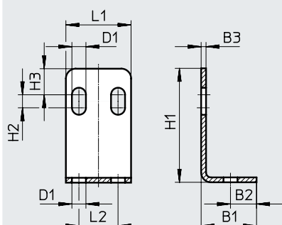
Escuadra de montaje HV-M5
