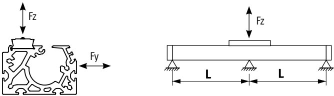
Fuerza Fz
